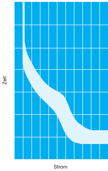
magnetisch-hydraulisch (HM)
