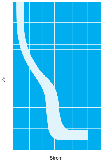
thermisch-magnetisch (TM)
